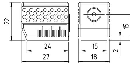
Рисунок 1 - эскиз преобразователя
