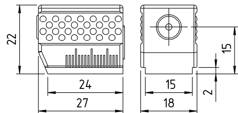
Рисунок 1 - эскиз преобразователя
