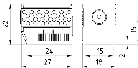
Рисунок 1 - эскиз преобразователя
